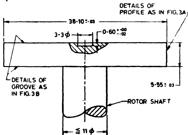
FIG. 4 ROTOR
